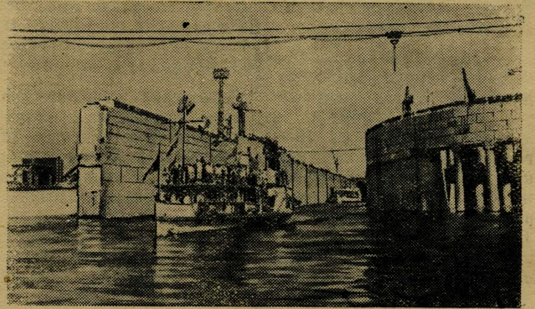
На строительстве Куйбышевской гидроэлектростанции состоялся пуск нижних судоходных шлюзов. На снимке: выход первых судов из камеры шлюза. Фото А. Батанова. Фотохроника ТАСС
