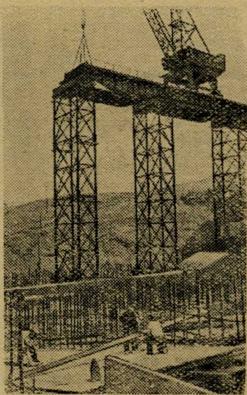
Таджикская ССР. Строительство Кайраккумской гидроэлектростанции на реке Сыр-Дарье. На снимке: монтаж секций бетонной эстакады на участке водосливной плотины. Фото В. Зайцева. Фотохроника ТАСС
